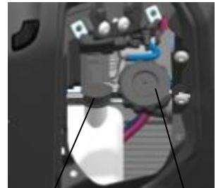
Δοχείο διαστολής Δοχείο ψυκτικού
